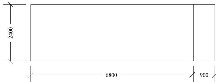
VIEW C (WALL)
